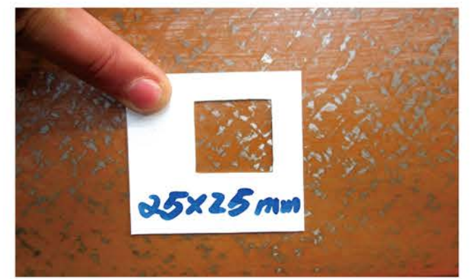
刮研检验
